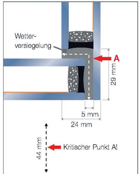
Fehlerhafte Fugentiefe bei 1K-Dichtstoff
