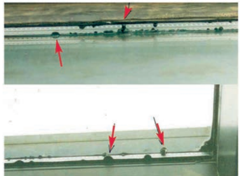
Auflösen der Butyl-Dichtung durch Migration
