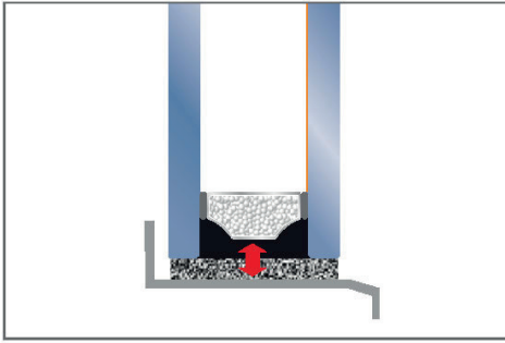
Wechselwirkung zwischen Randverbund und Klotz
