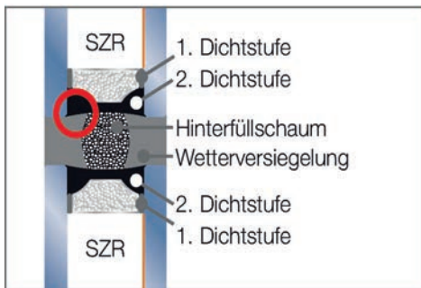
Wetterversiegelung in einem Isolierglasstoß
