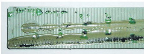
Klotz nach schädlichen Wechselwirkungen
